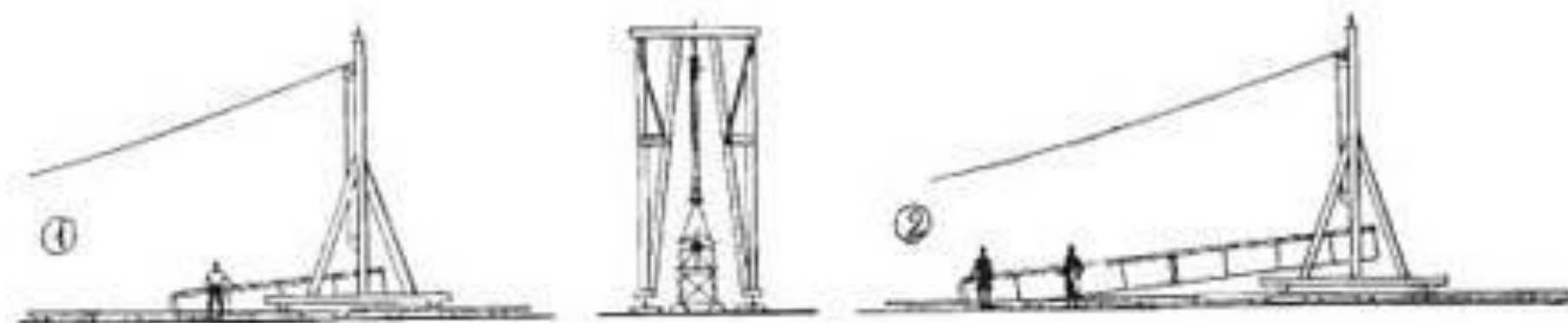
Montage des vereinfachten Abschluß-Katapultes
